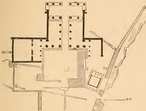
FIG. 24. — PLAN DES PROPYLÉES DE L'ACROPOLE D'ATHÈNES.
